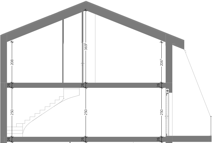
COUPE AA
